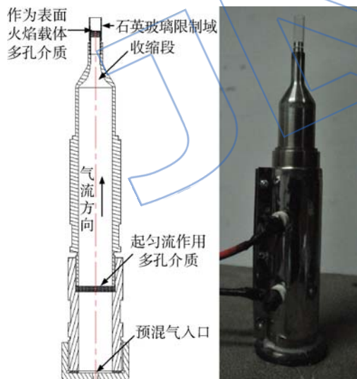
图 2 实验段简图和实物图
