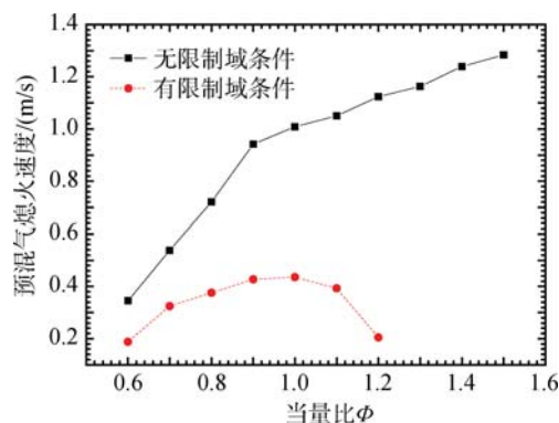
图5 有/无限制域,表面火焰预混气熄火速度
